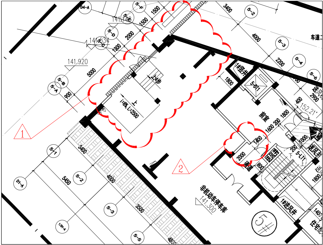
局部地下一层平面图 变更前
