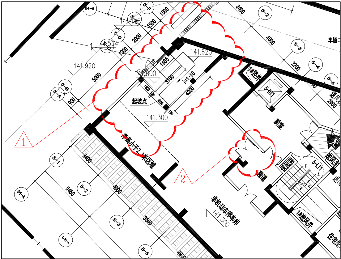
局部地下一层平面图 变更后
