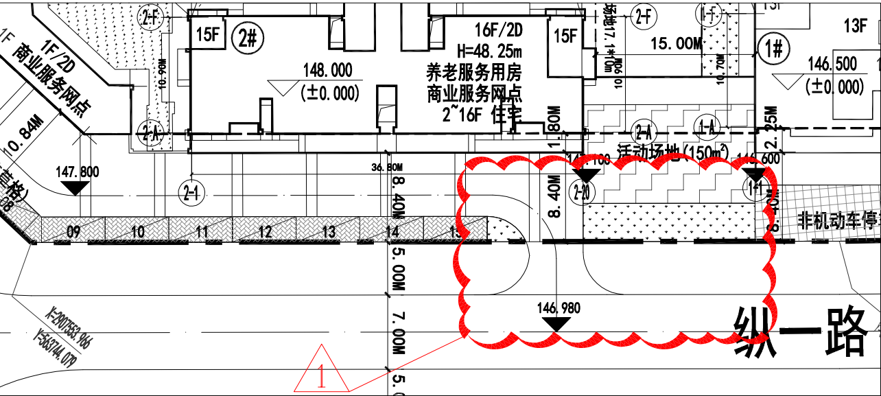
局部总平面图 变更前
