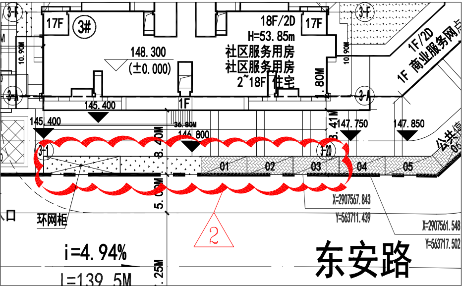
局部总平面图 变更前
