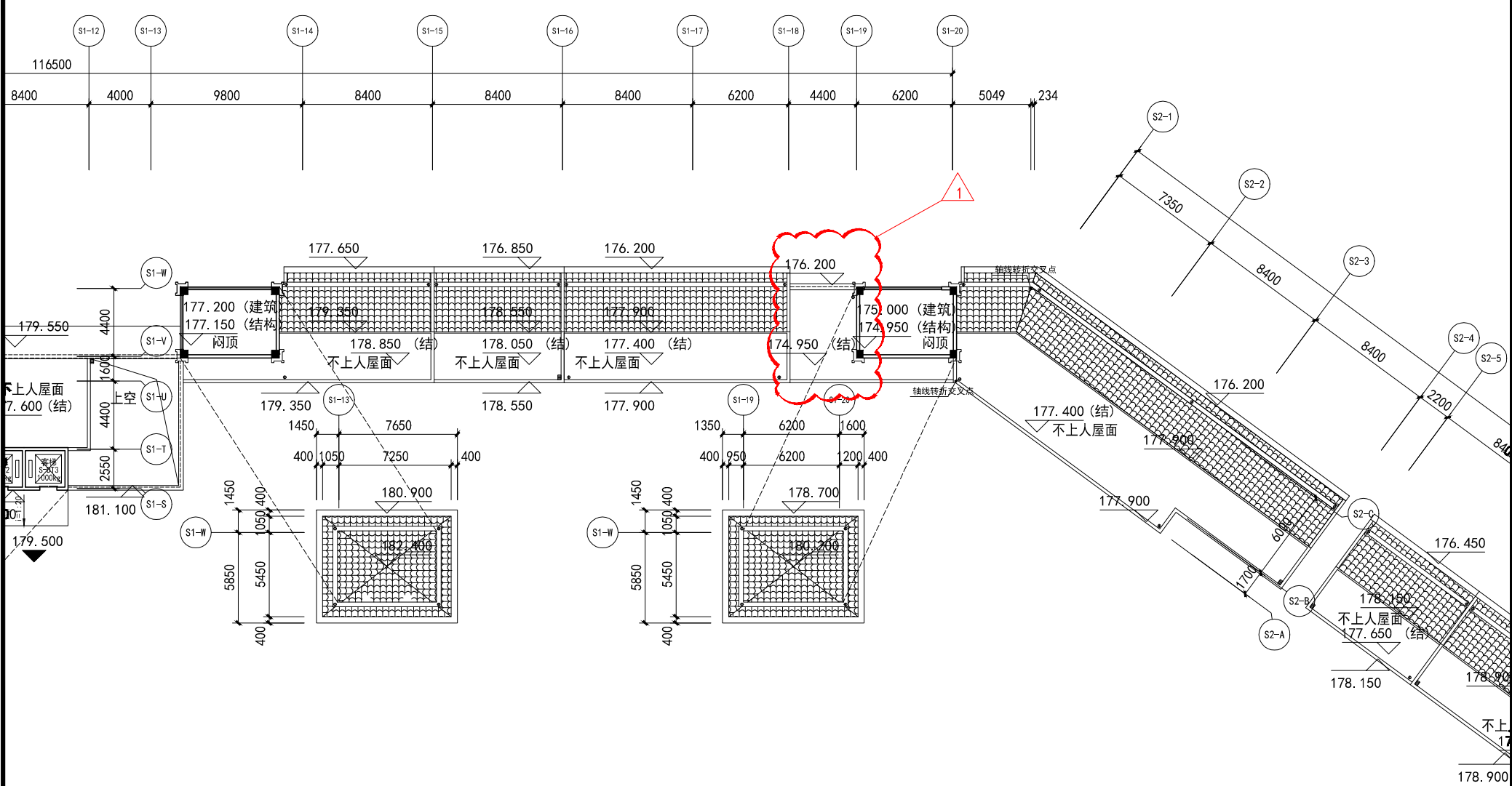
沿街商业屋面层平面图(S1-18轴~S1-19轴) 1:250
