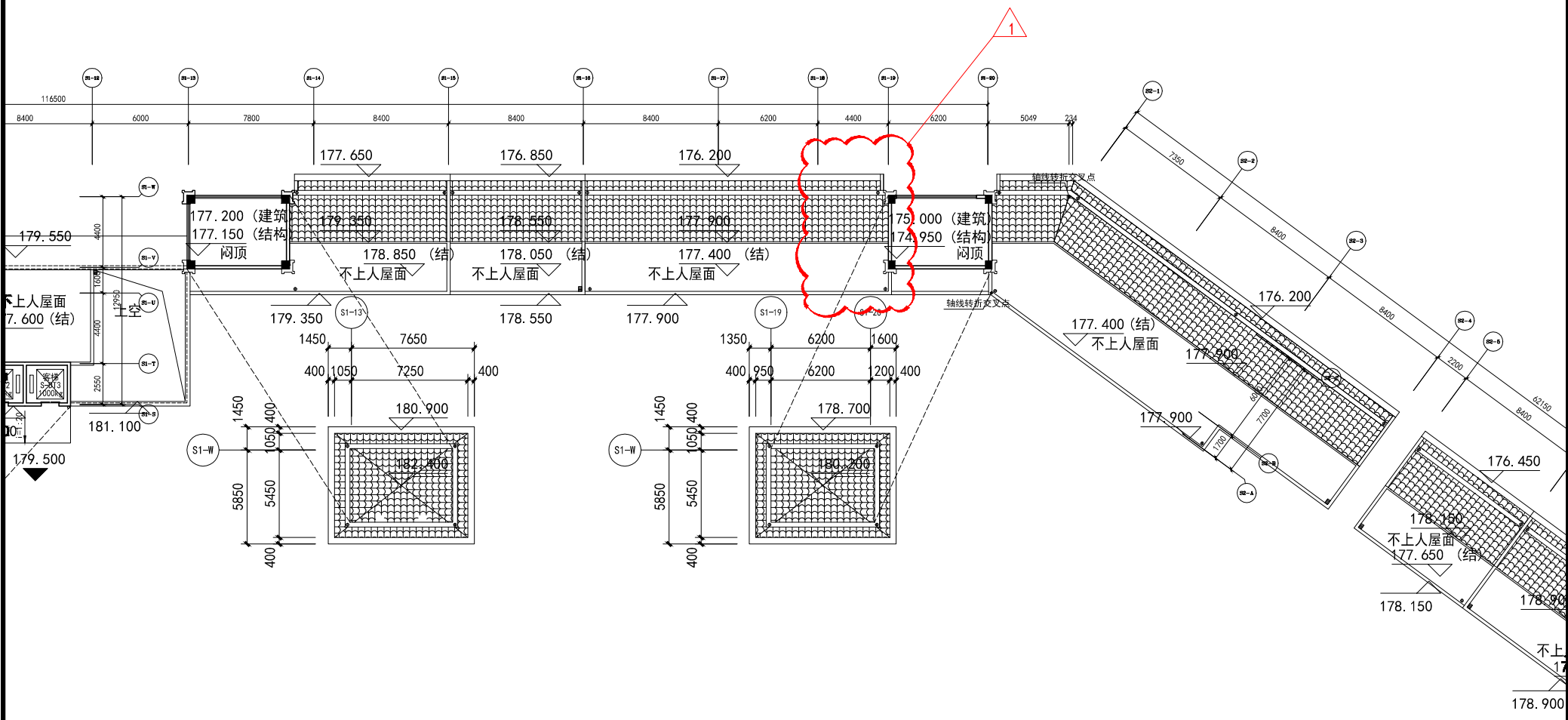
沿街商业屋面层平面图(S1-18轴~S1-19轴) 1:250
