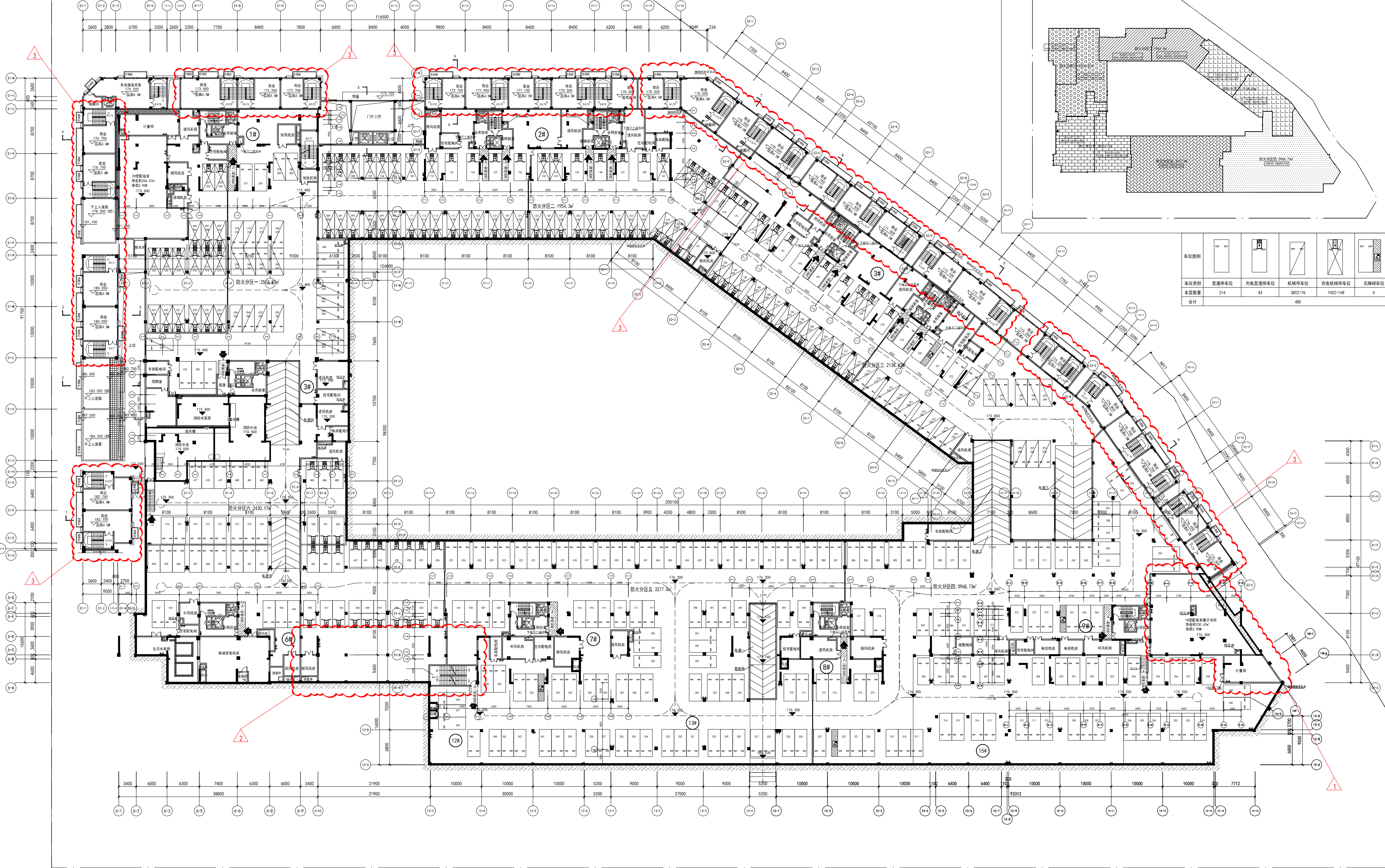
地下一层平面图 1:500
