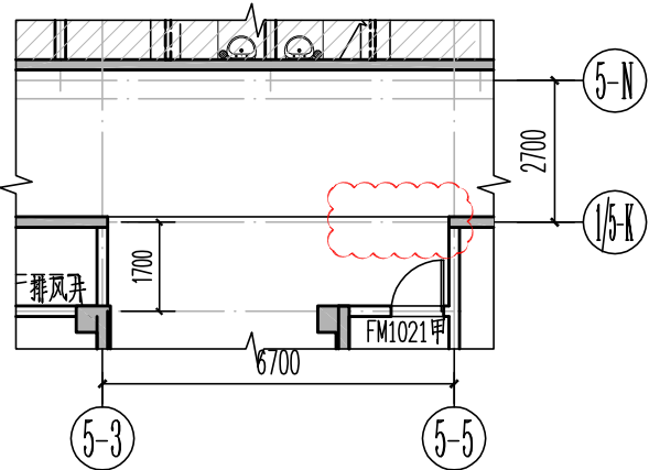
修改前地下室局部平面图一
