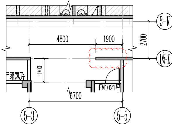
修改后地下室局部平面图一
