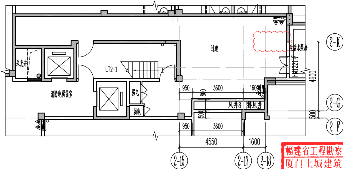
修改前地下室局部平面图二
