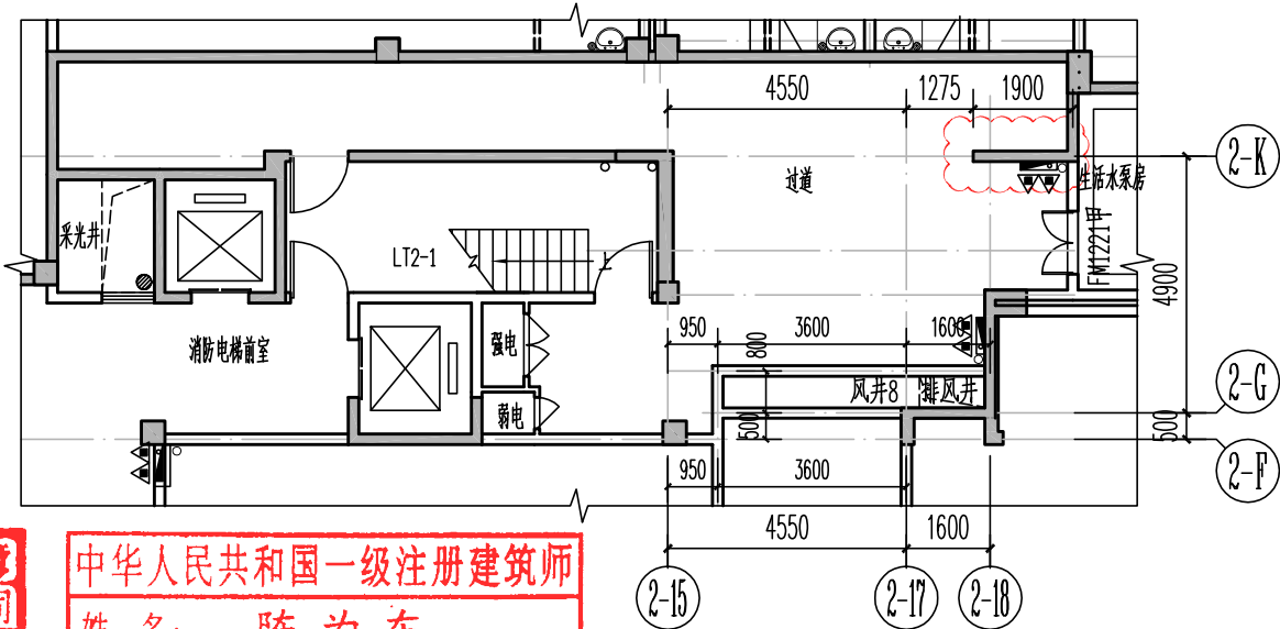
修改后地下室局部平面图二
