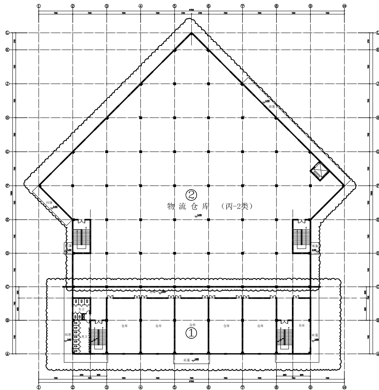
变更前二层平面方案 1:100 \nabla 3.600 本层建筑面积: 3165.94m 2
