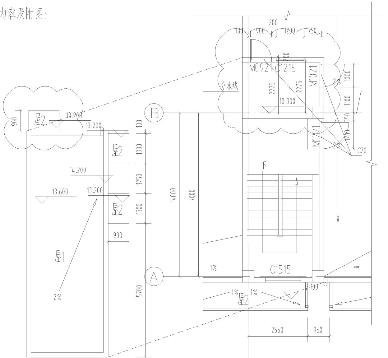
屋顶局部平面图 1:100 变更后
