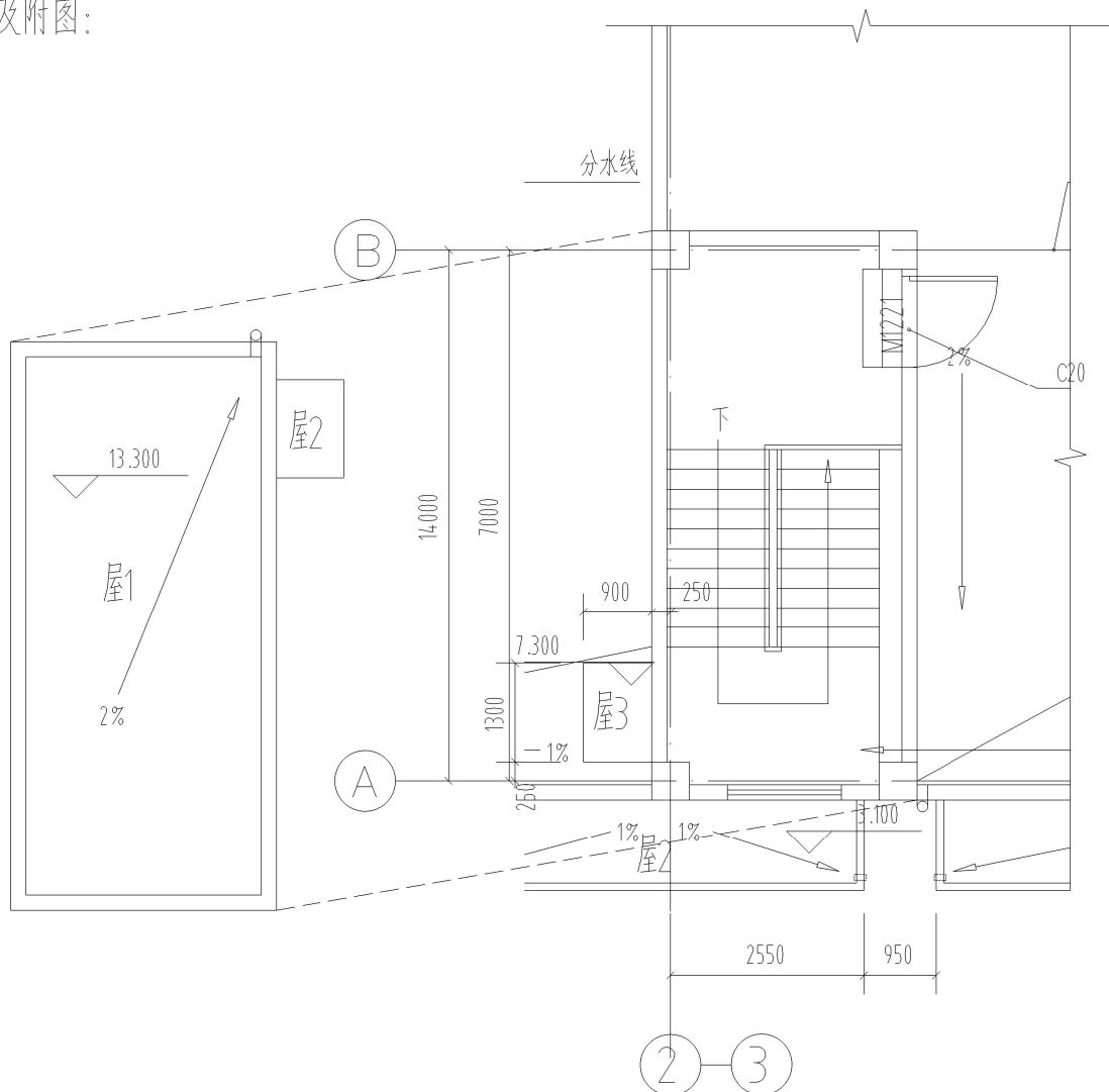
屋顶局部平面图 1:100
