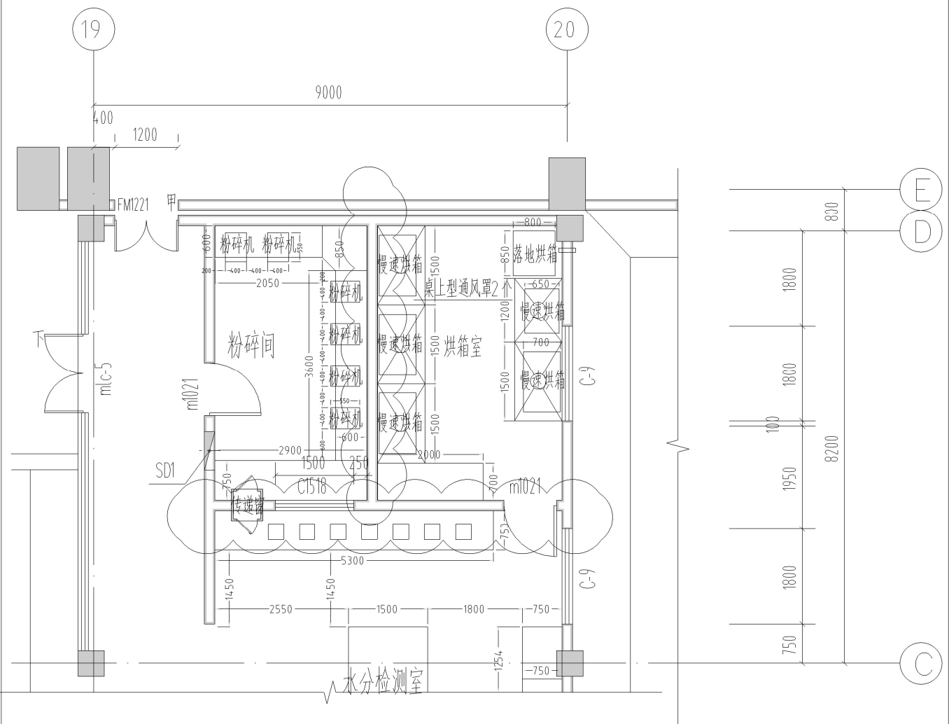
联合工房 I 区一层平面图 变更后
