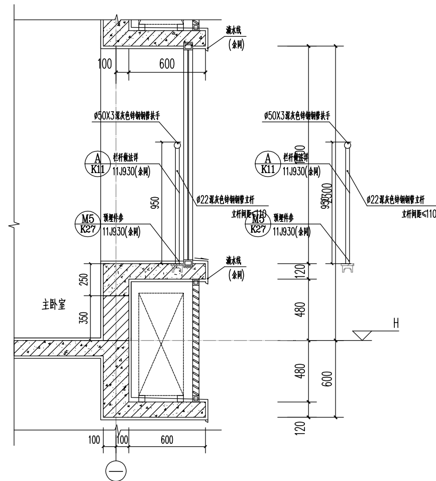
飘窗大样
