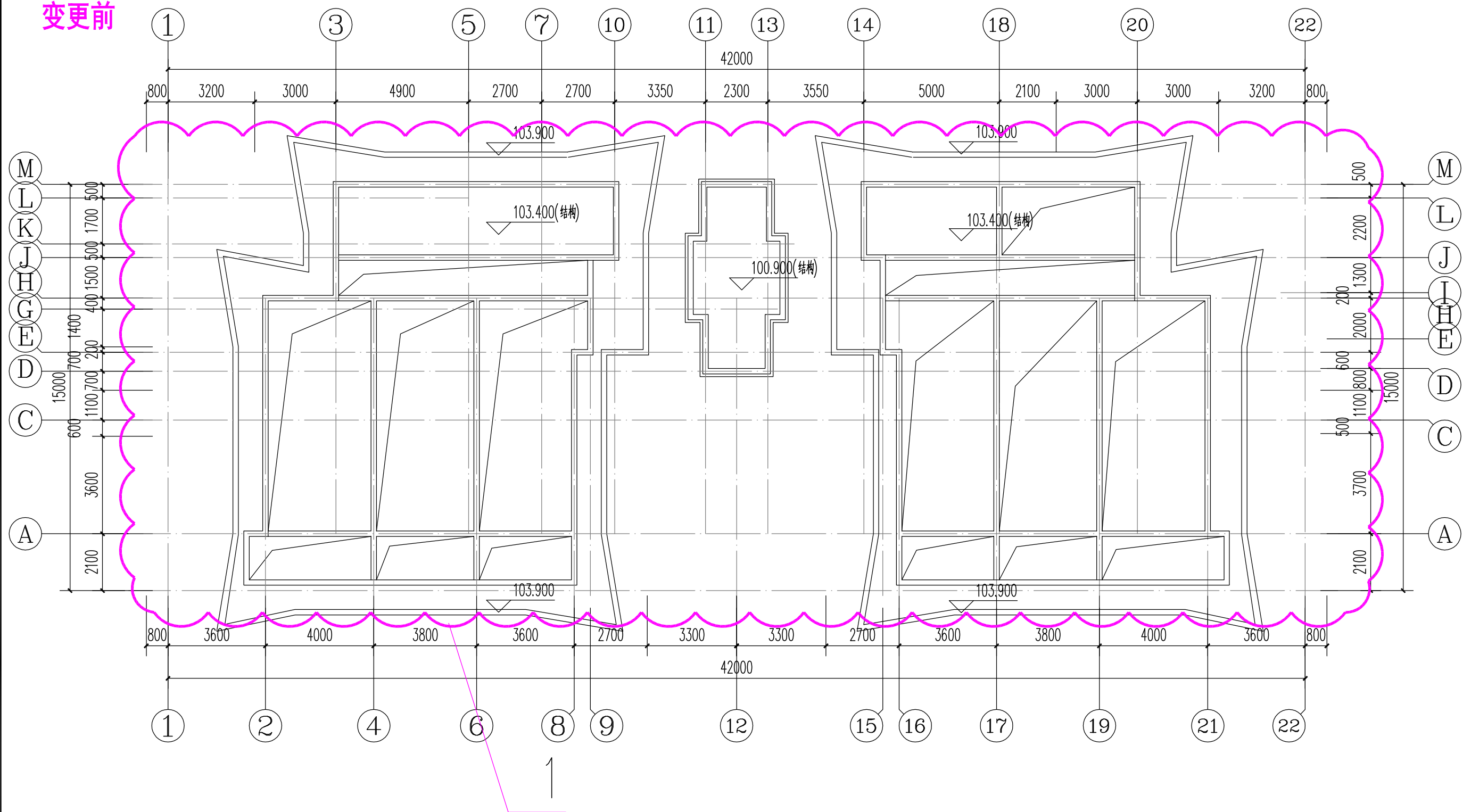
12#屋顶构架平面图
