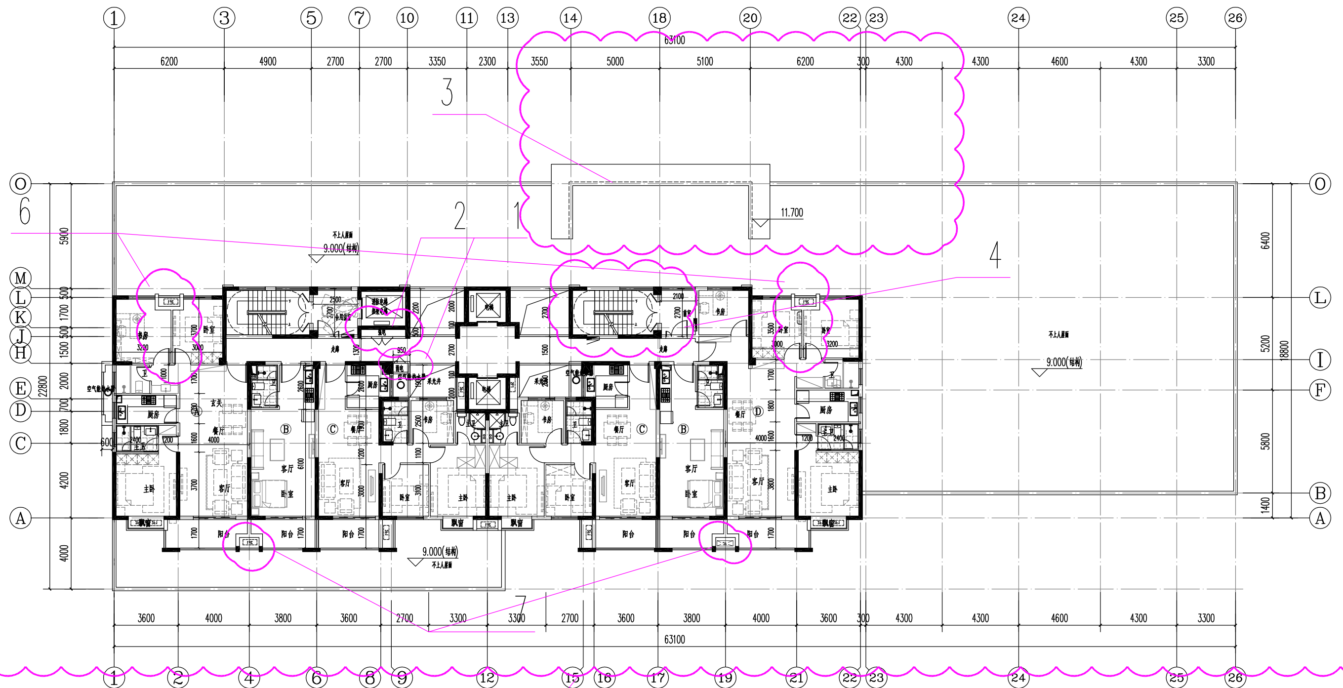
12井三层平面图
