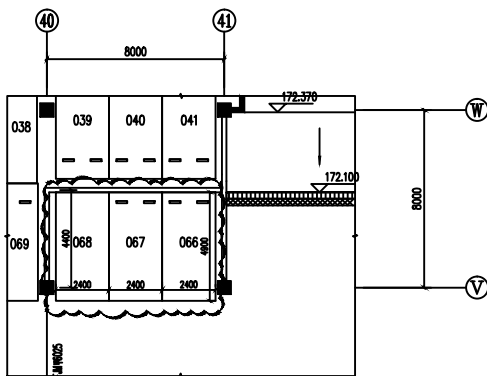
地下室负一层局部车位变更图三 (变更后)
