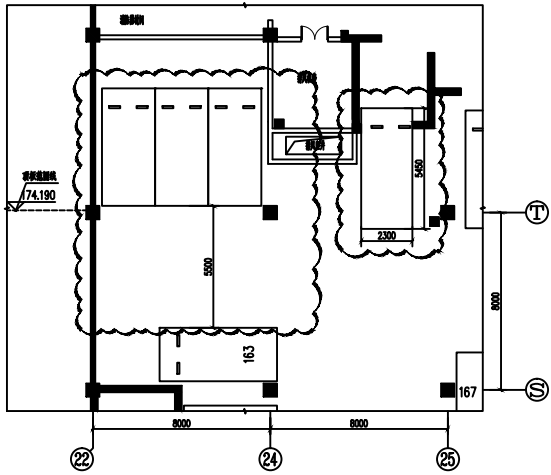
地下室负一层局部车位变更图一 (变更后)
