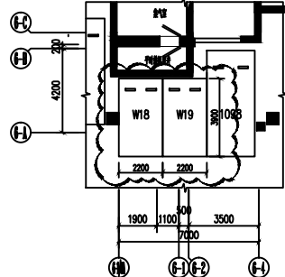
地下室负二层局部车位变更图一 (变更后)
