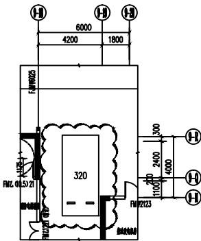
地下室负一层局部车位变更图四 (变更前)
