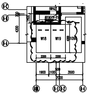
地下室负二层局部车位变更图一 (变更前)
