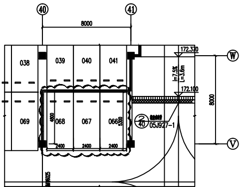
地下室负一层局部车位变更图三 (变更前)
