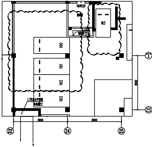
地下室负一层局部车位变更图一 (变更前)
