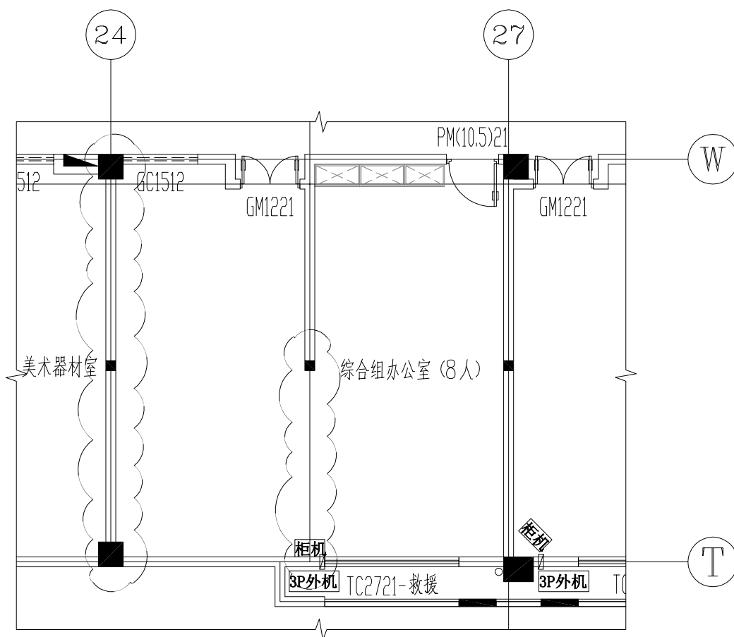
变更后三层局部平面图
