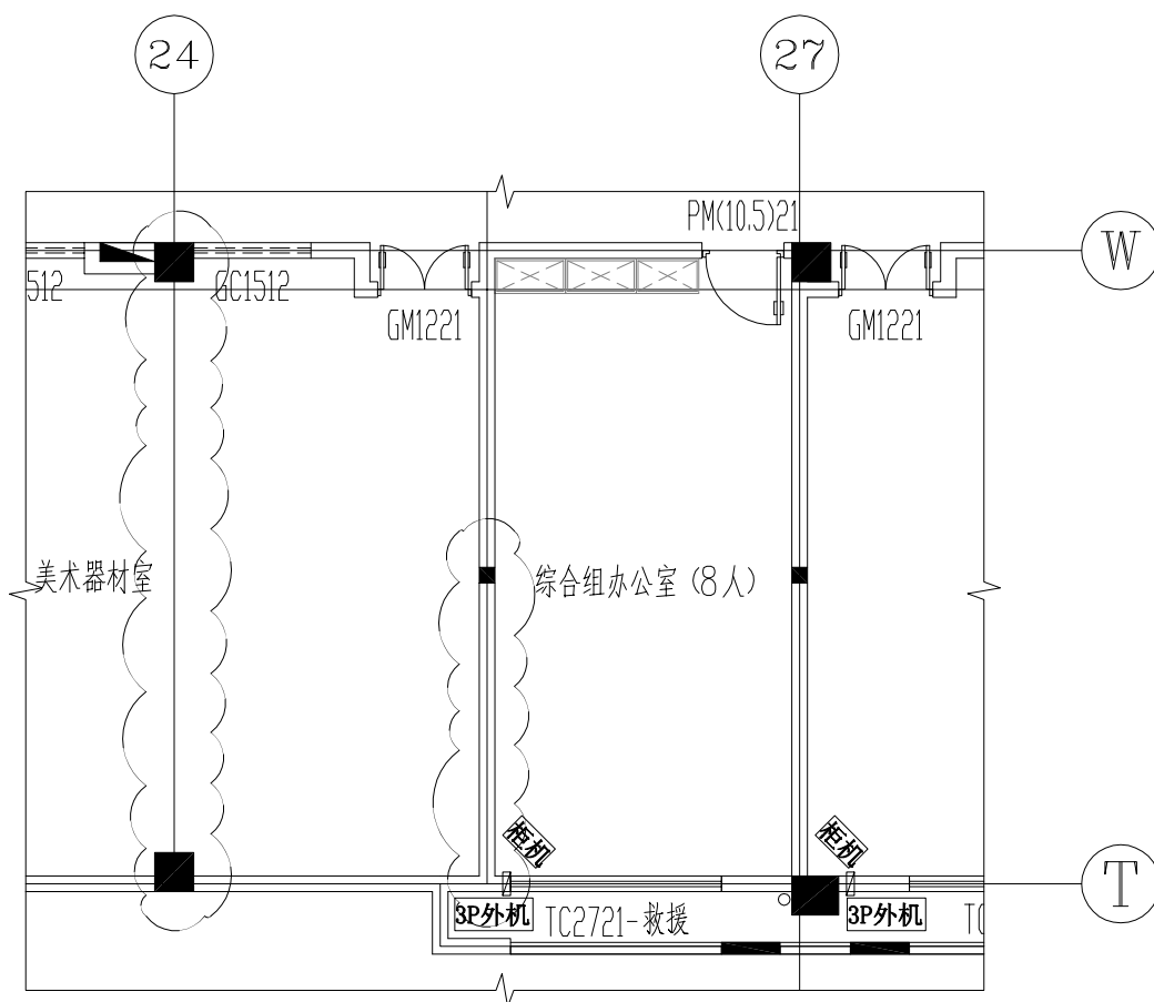
变更前三层局部平面图
