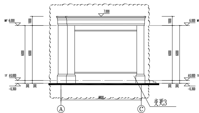
①~③轴立面图 (修改后) 1:100
