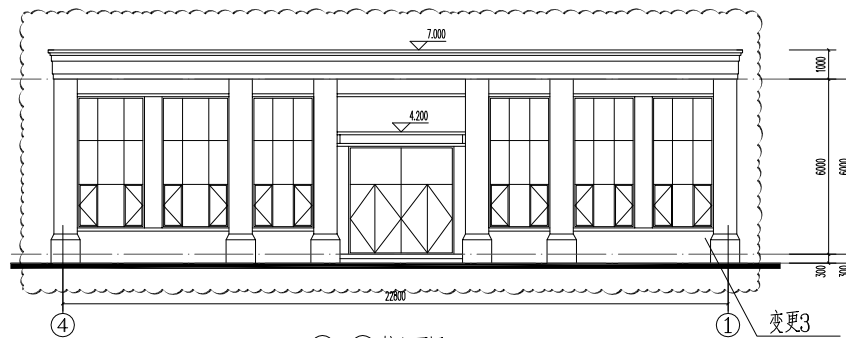
④~①轴立面图 (修改后) 1:100
