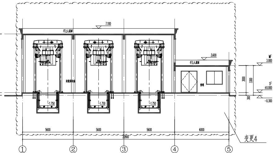
1-1剖面图 (修改前) 1:100
