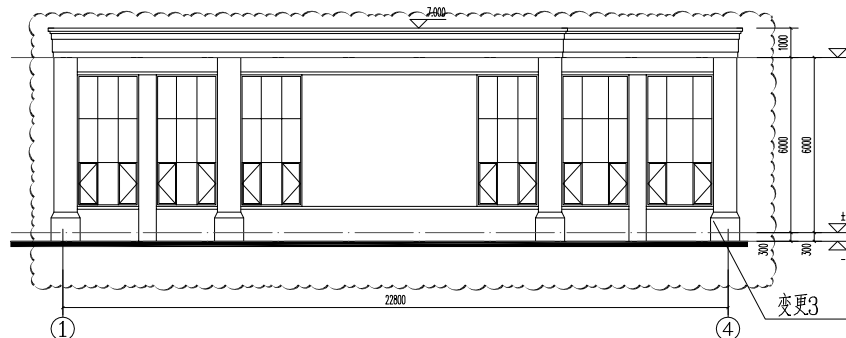
①~④轴立面图 (修改后) 1:100
