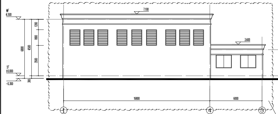
①~⑤轴立面图 (修改前) 1:100
