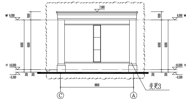
③~①轴立面图 (修改后) 1:100
