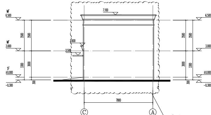
③~①轴立面图 (修改前) 1:100
