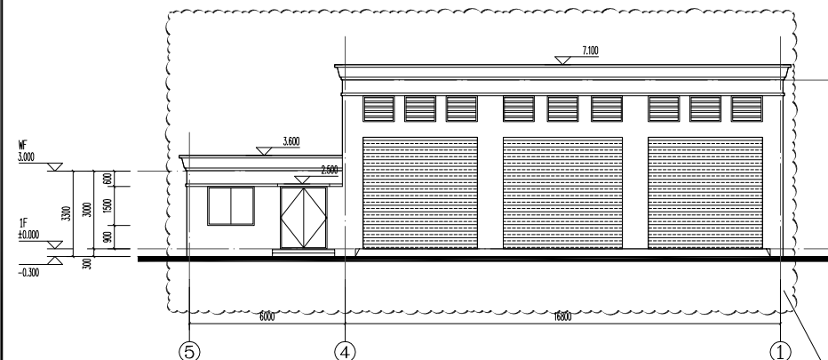
⑤~①轴立面图 (修改前) 1:100
