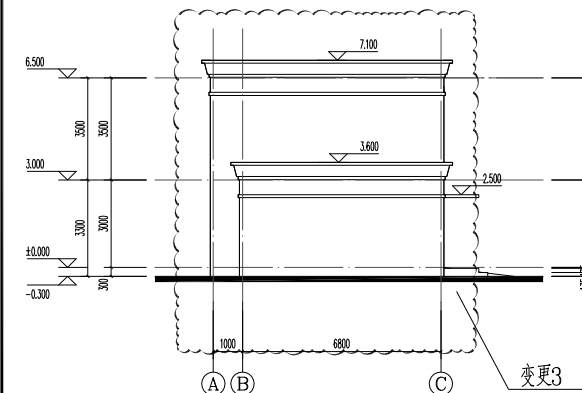
①~③轴立面图 (修改前) 1:100
