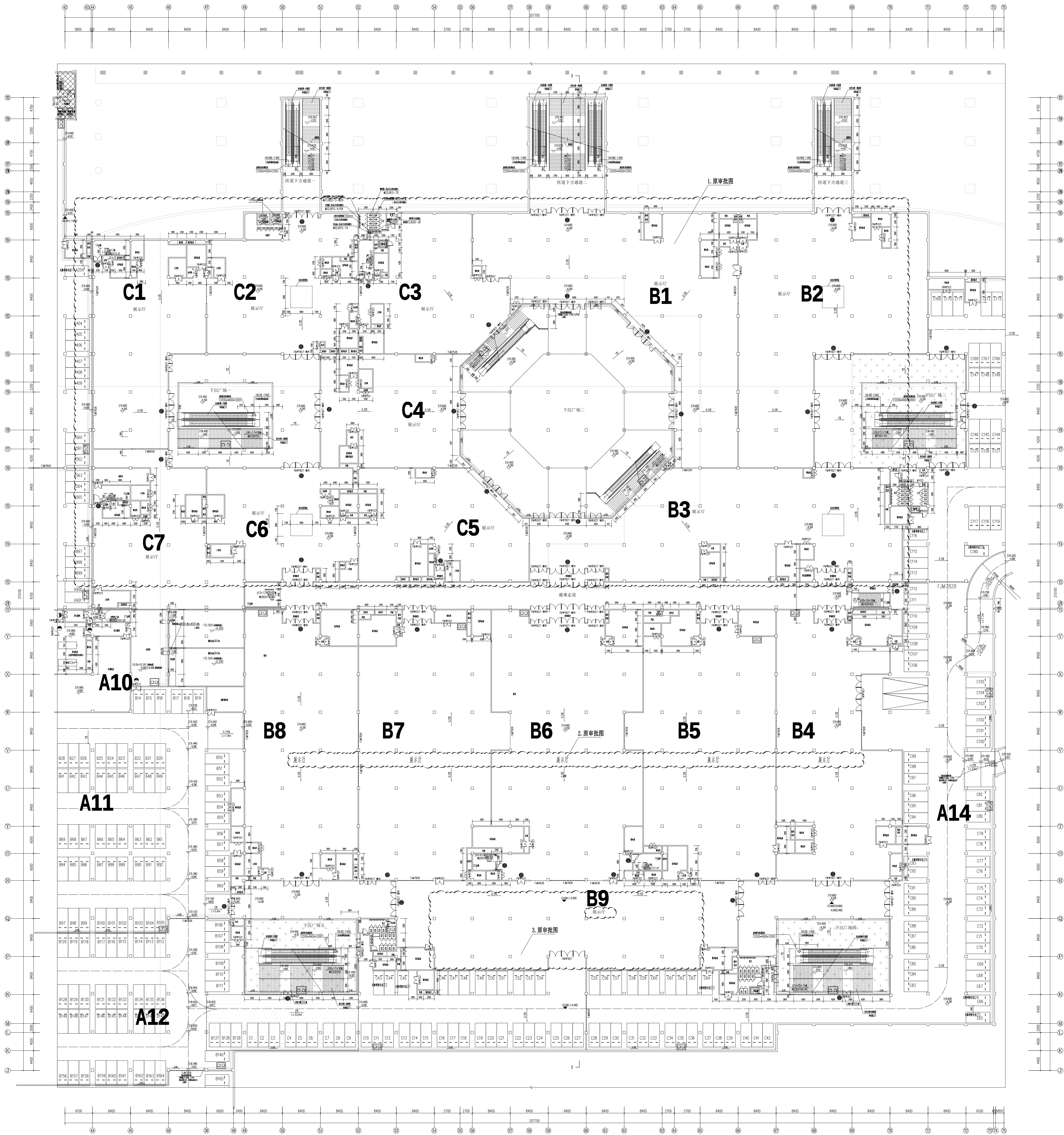
地下室局部平面图 (原审批图)
