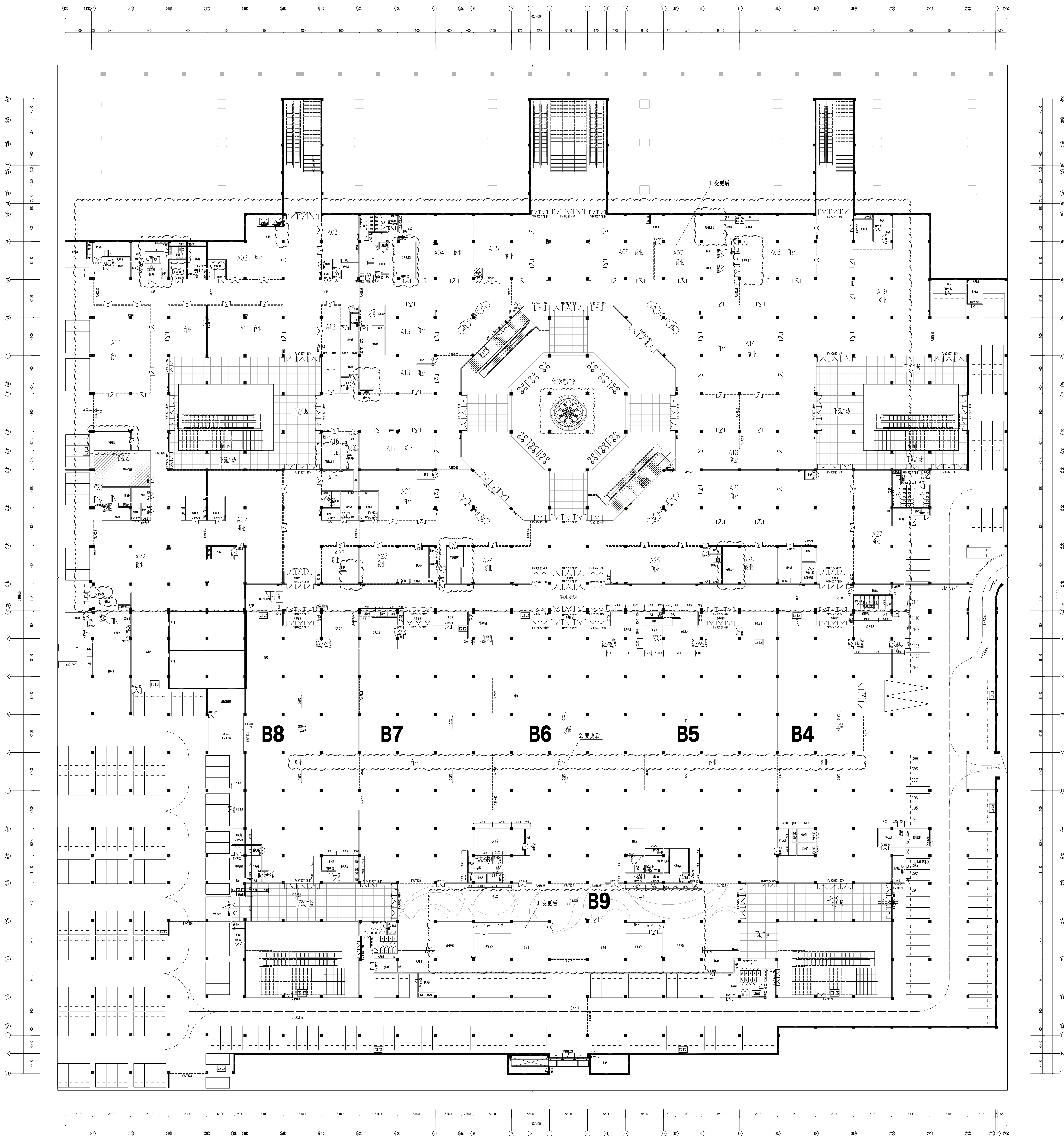
地下室局部平面图 (变更后)
