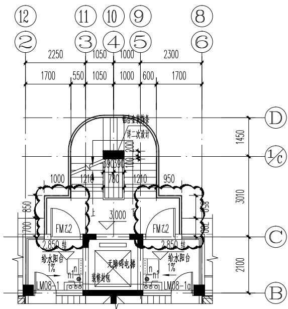
二层局部平面图(修改后) 1:100
