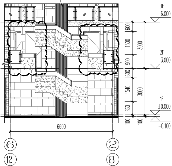
⑬~①轴局部立面图(修改后) 1:100
