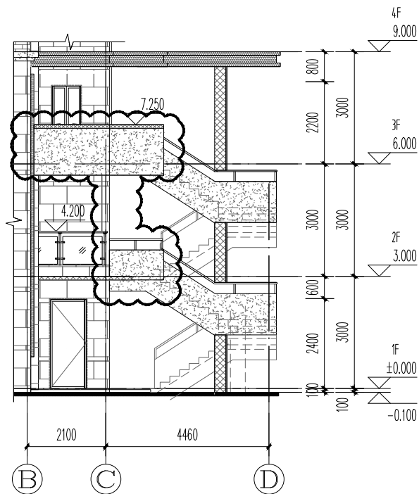
①~④轴局部立面图(修改后) 1:100
