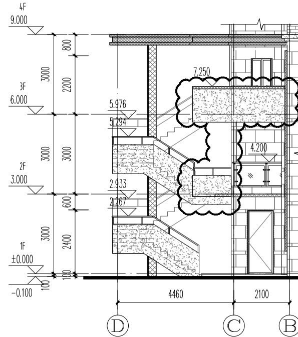
④~①轴局部立面图(修改后) 1:100
