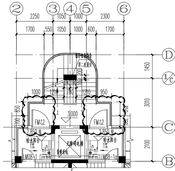
二层局部平面图(修改后) 1:100
