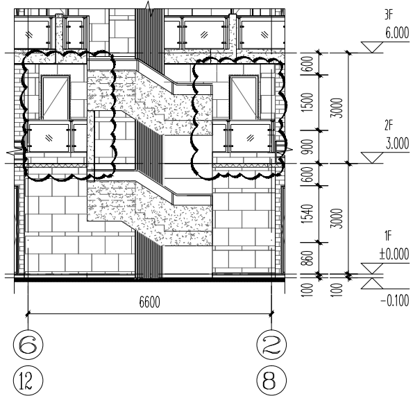
⑬~①轴局部立面图(修改前) 1:100
