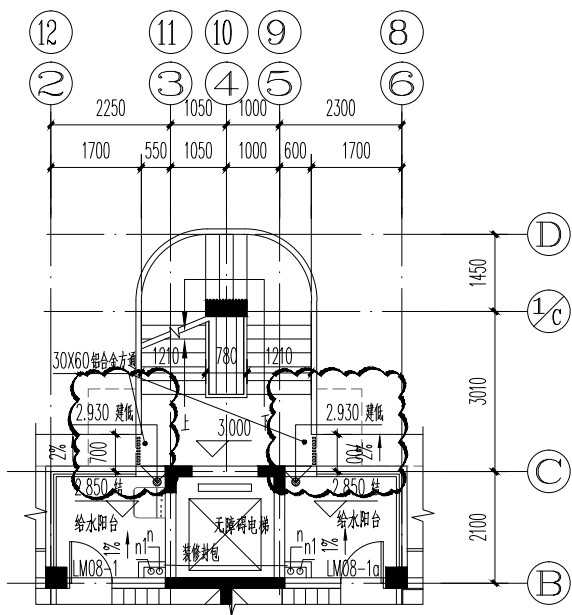
二层局部平面图(修改前) 1:100
