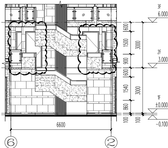
⑦~①轴局部立面图(修改后) 1:100
