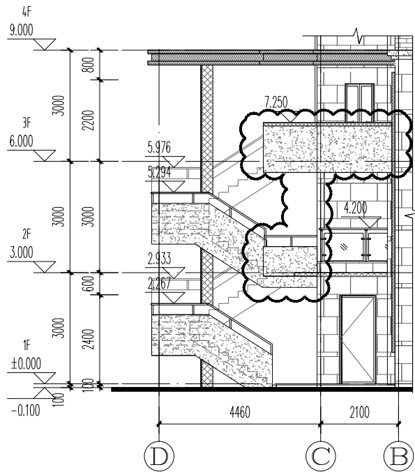
①~④轴局部立面图(修改后) 1:100
