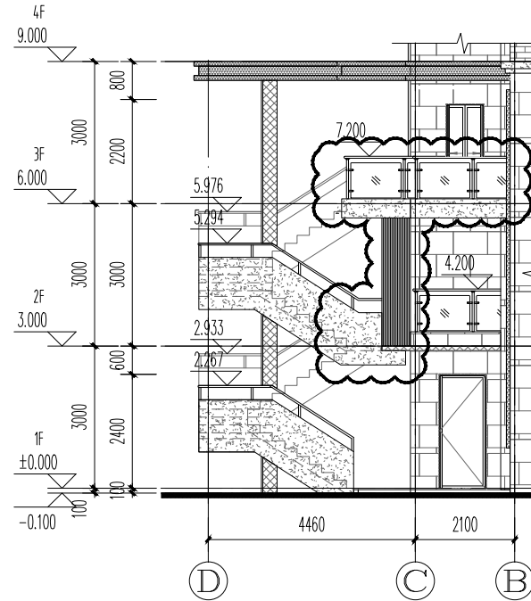
④~①轴局部立面图(修改前) 1:100
