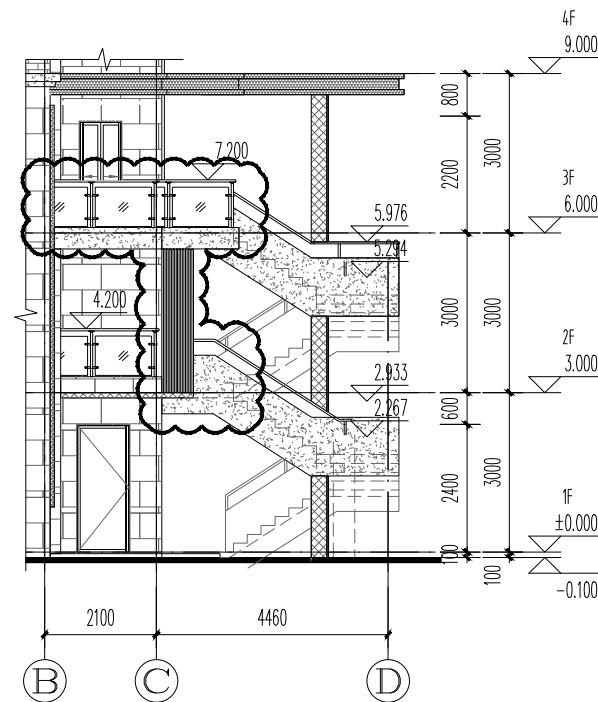
①~④轴局部立面图(修改前) 1:100
