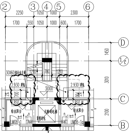
二层局部平面图(修改前) 1:100
