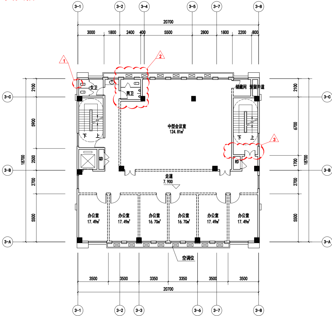
三层平面图 1:150
