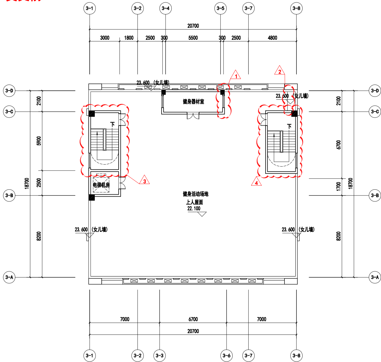
屋顶平面图 1:150
