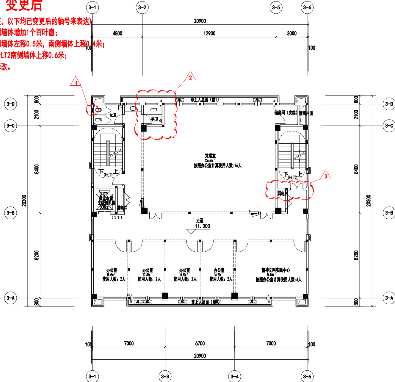
四层平面图 1:150
