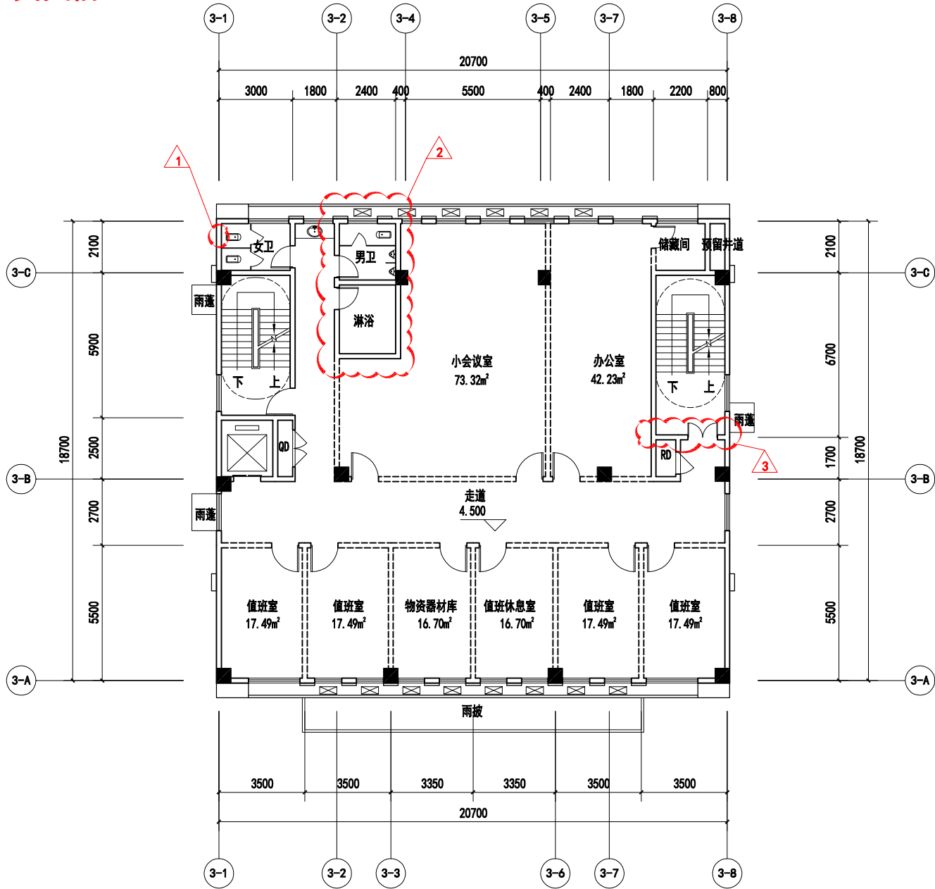
二层平面图 1:150 本层计容面积: 395.01m²
