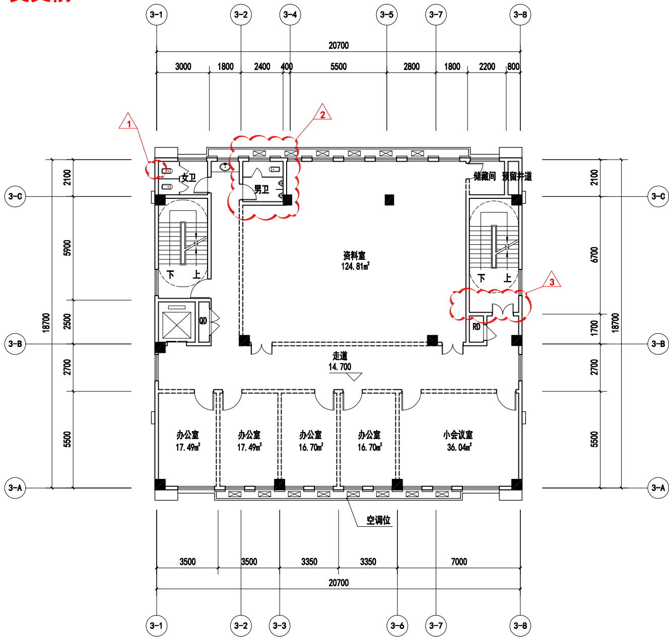
五层平面图 1:150
