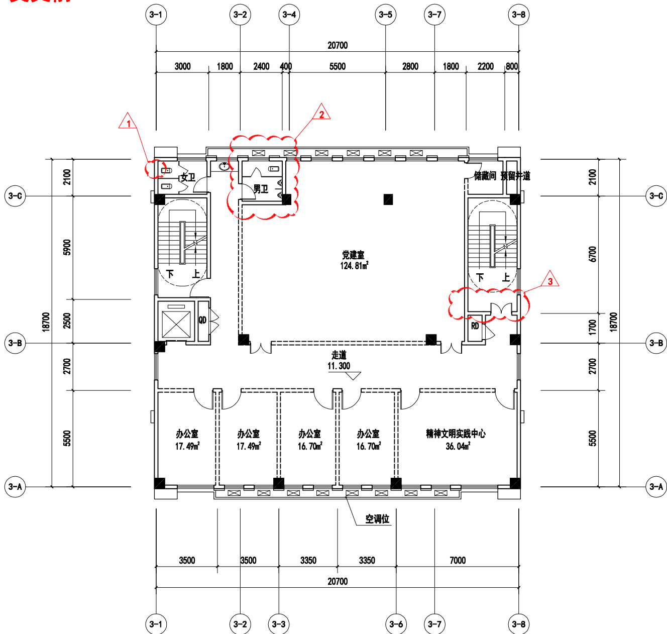
四层平面图 1:150
