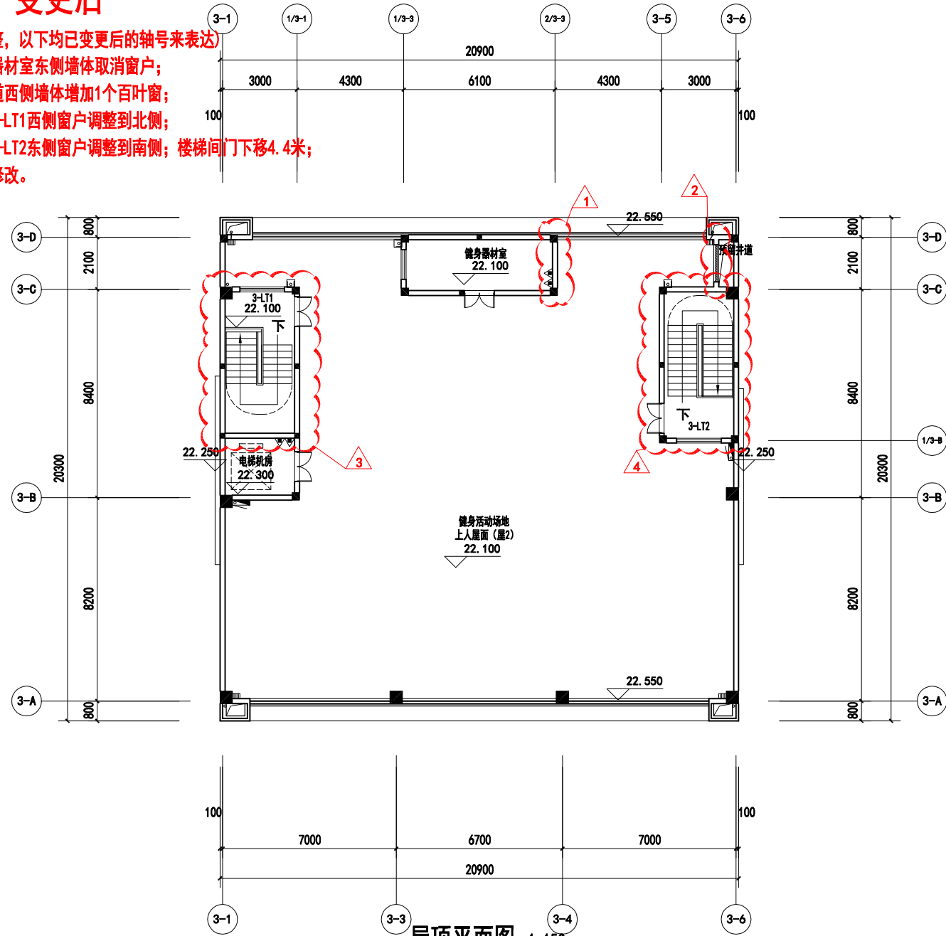
屋顶平面图 1:150
