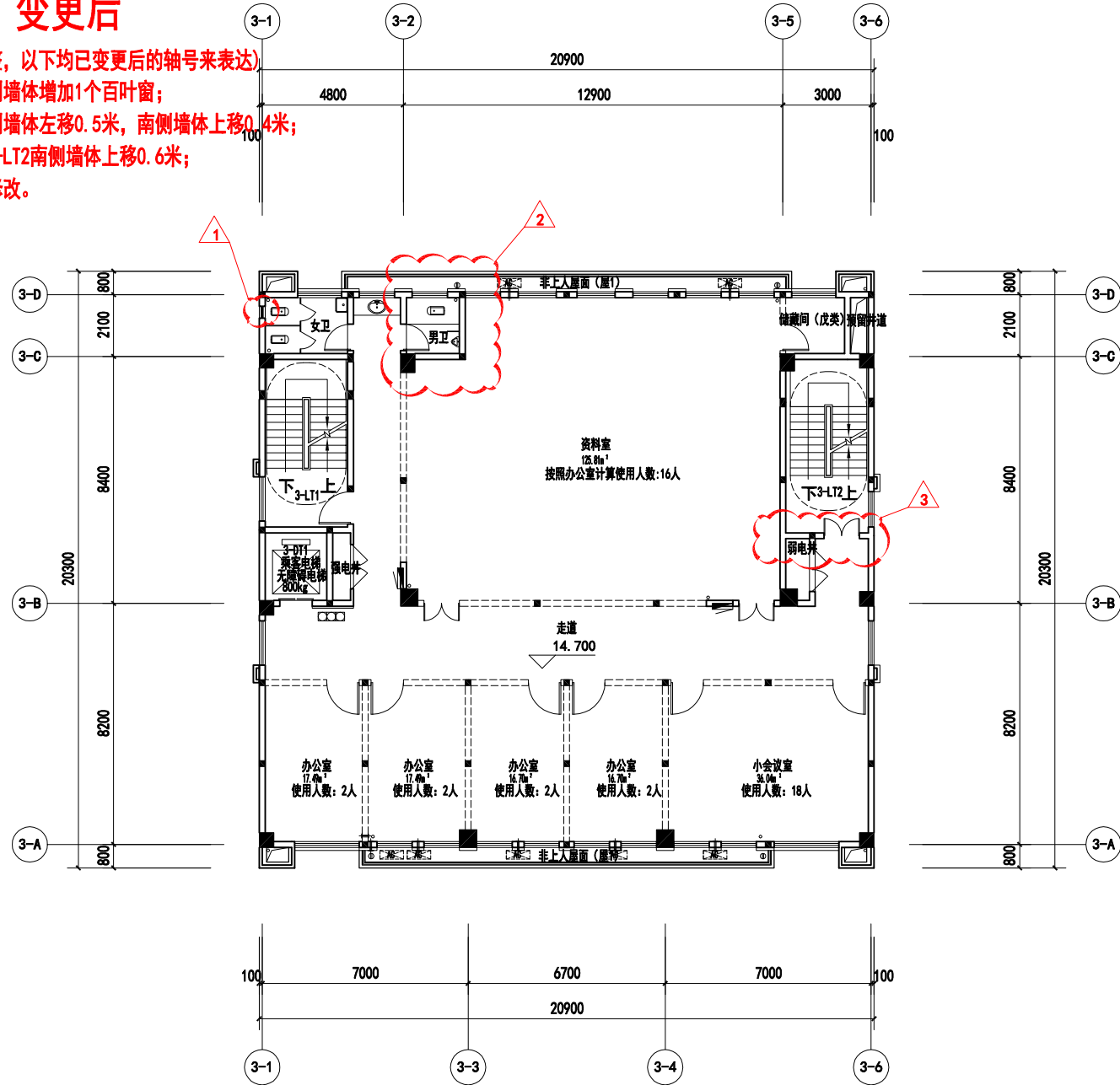
五层平面图 1:150
