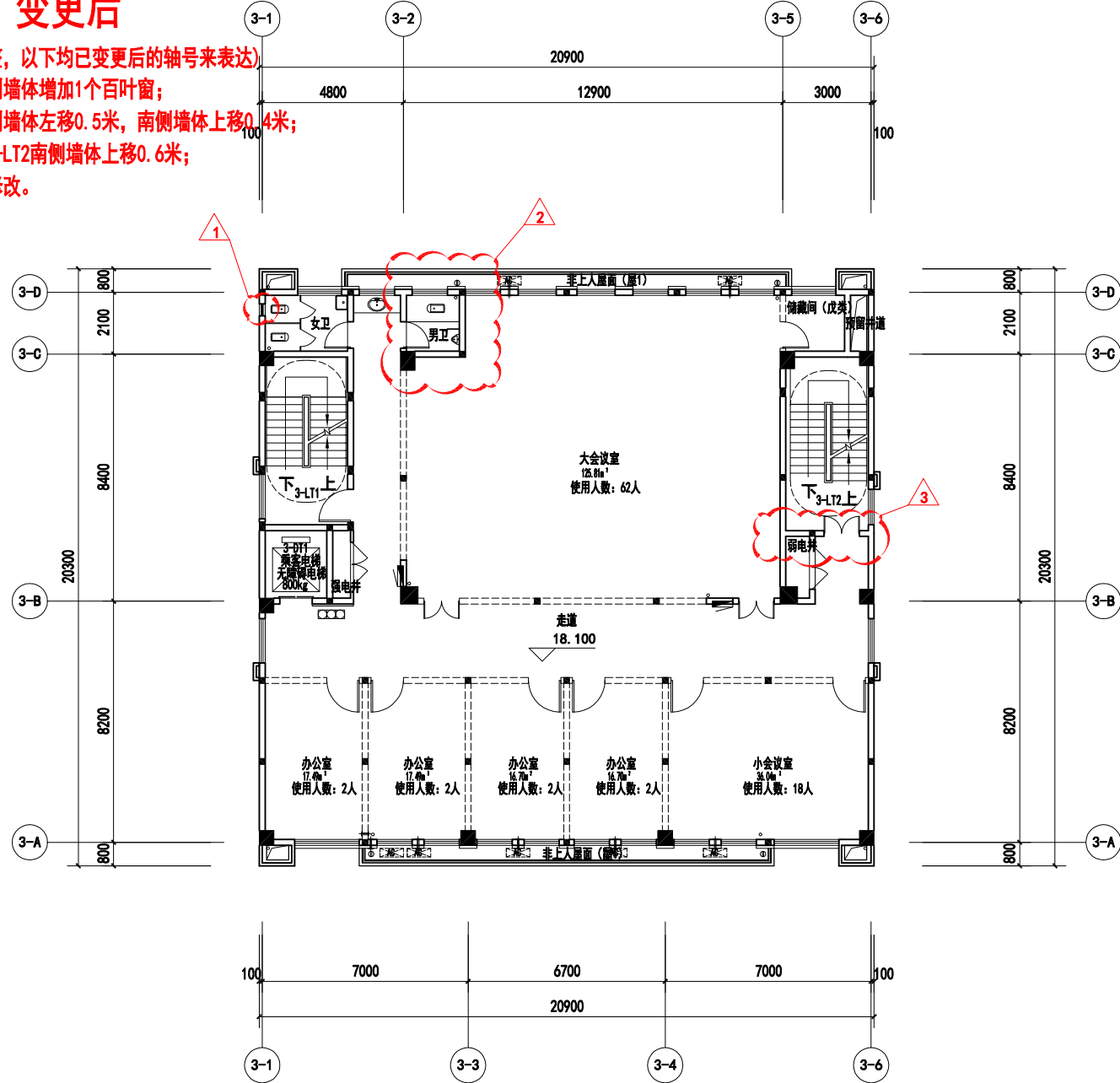
六层平面图 1:150 本层计客面积: 395.01m²
