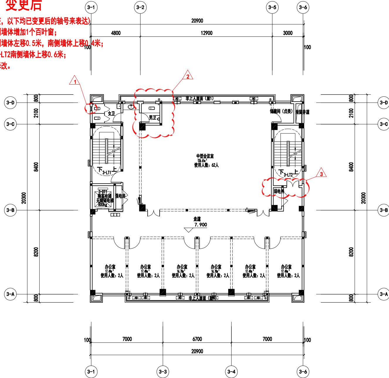
三层平面图 1:150
