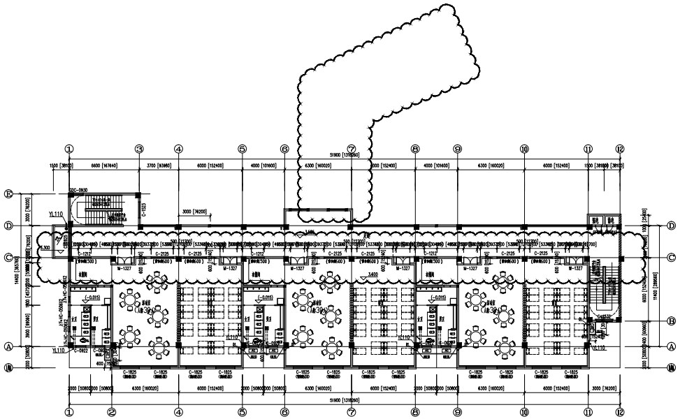
二层平面图(变更后) 1:100
