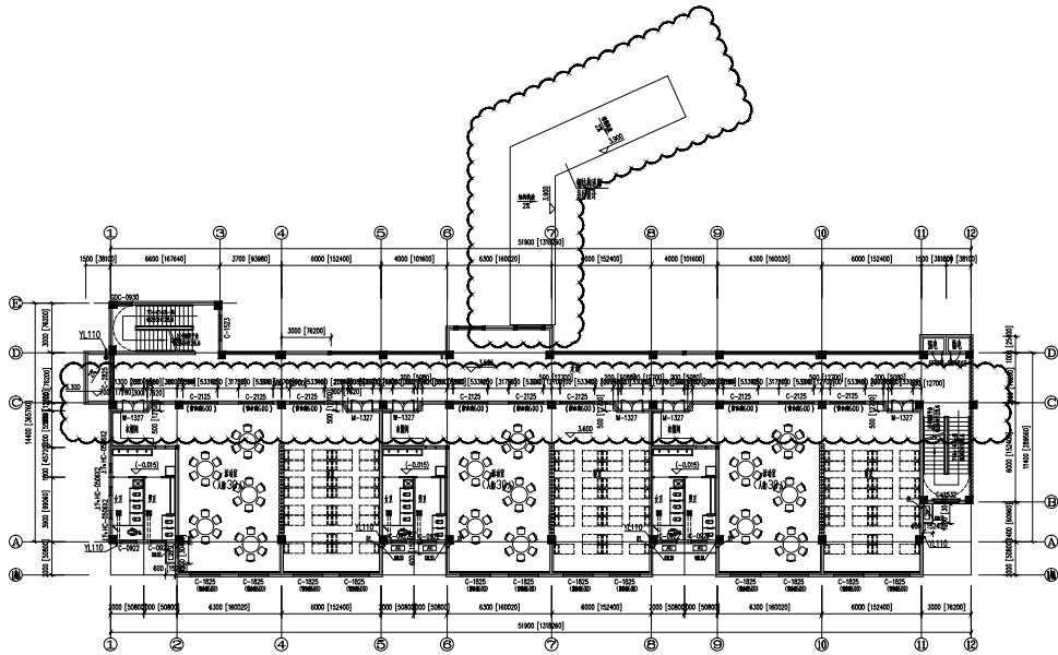
二层平面图(原图) 1:100
