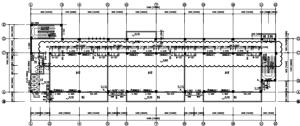
四层平面图 (变更后) 1:100
