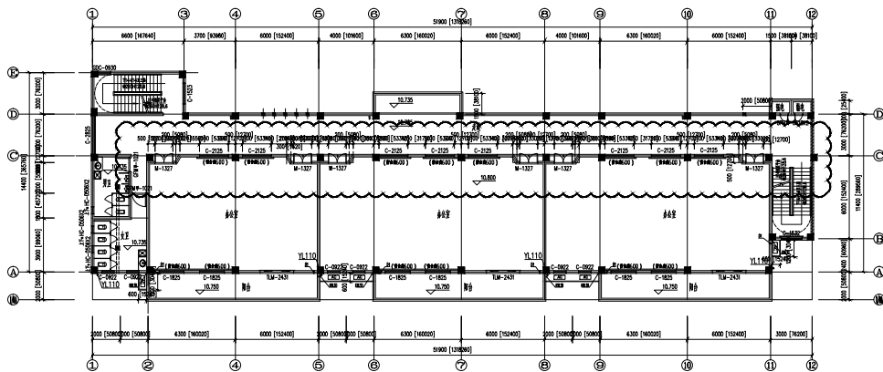
四层平面图 (原图) 1:100
