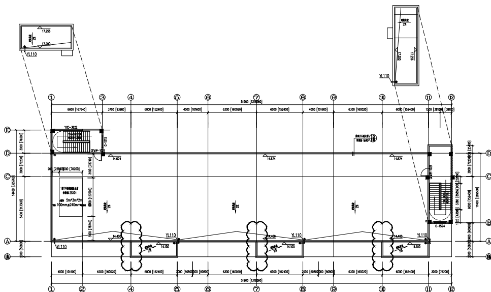
屋面平面图 (原图) 1:100
