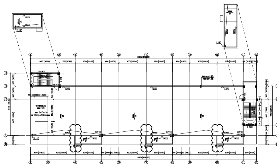
屋面平面图 (变更后) 1:100
