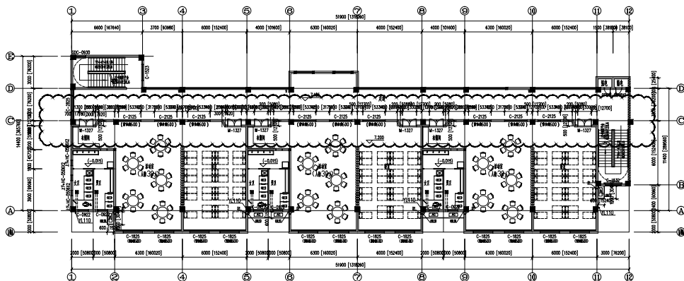
三层平面图 (原图) 1:100
