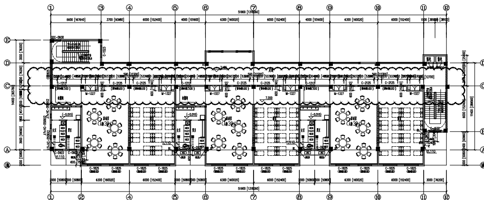
三层平面图 (变更后) 1:100
