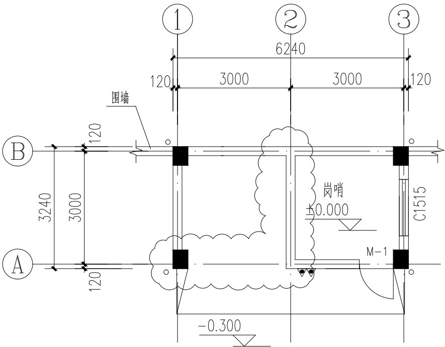
岗哨一层平面图 1:100 (变更前)
