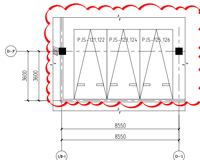
地下一层局部平面图二 (变更后)
