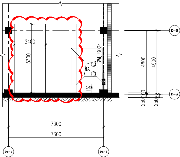
地下一层局部平面图一(变更前)
