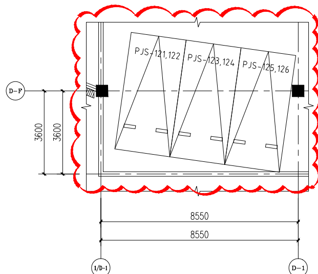
地下一层局部平面图二 (变更前)
