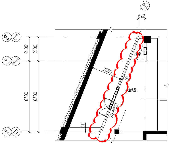
地下一层局部平面图二 (变更前)
