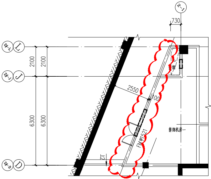
地下一层局部平面图二 (变更后)
