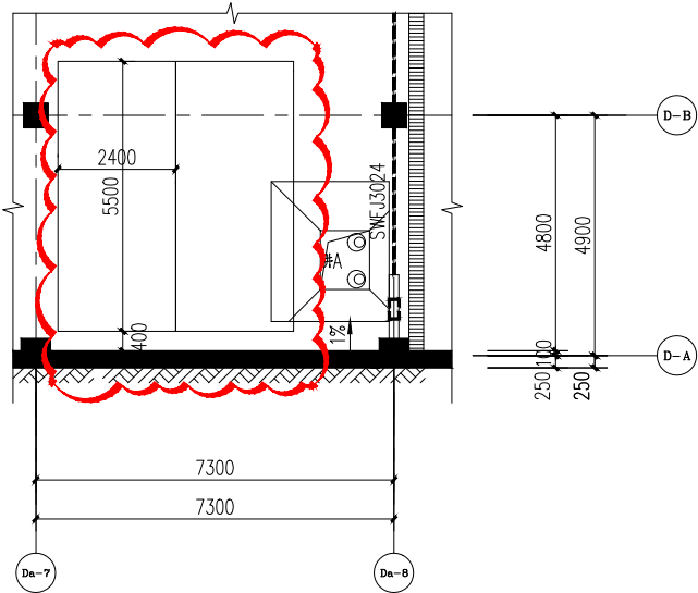
地下一层局部平面图一(变更后)
