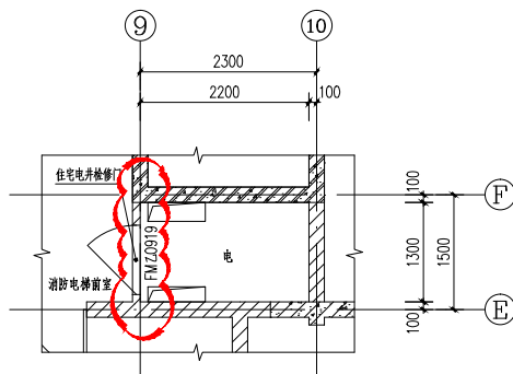
二至六层局部平面图(变更前)
