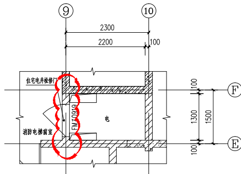
二至六层局部平面图(变更后)
