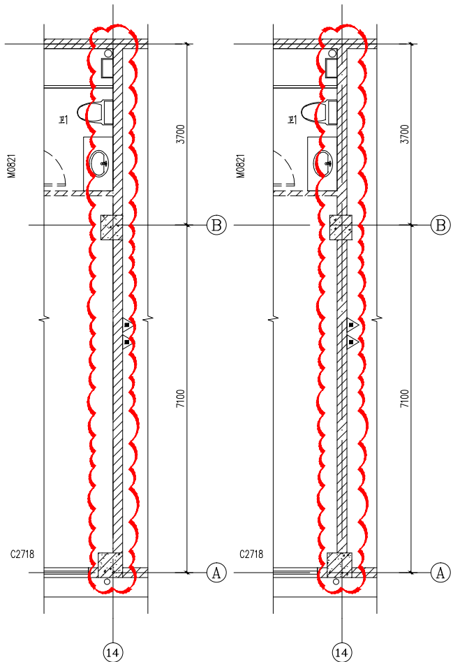
三层局部平面图(变更前)
